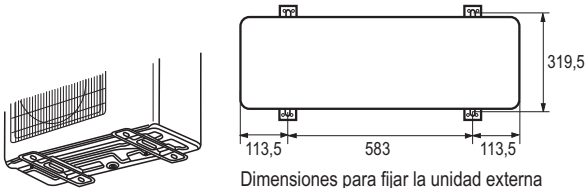
Dimensiones para fijar la unidad externa al piso. Unidades en mm Sistemas de 24 000 BTU/h de capacidad
