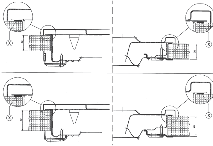
Fijación frontal
